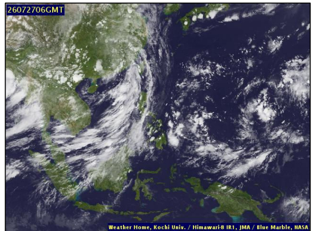
ภาพถ่ายดาวเทียม วันที่ ๒๗ ก.ค. ๒๕๖๙ เวลา ๑๓.๐๐ น.
