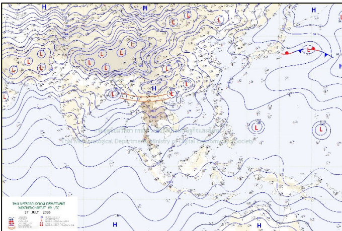
แผนที่อากาศ วันที่ ๒๗ ก.ค. ๒๕๖๙ เวลา ๐๗.๐๐ น.
